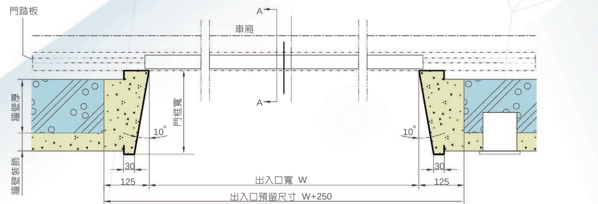
B-B 斷面
