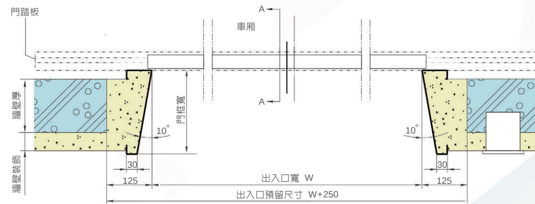
B-B 斷面
