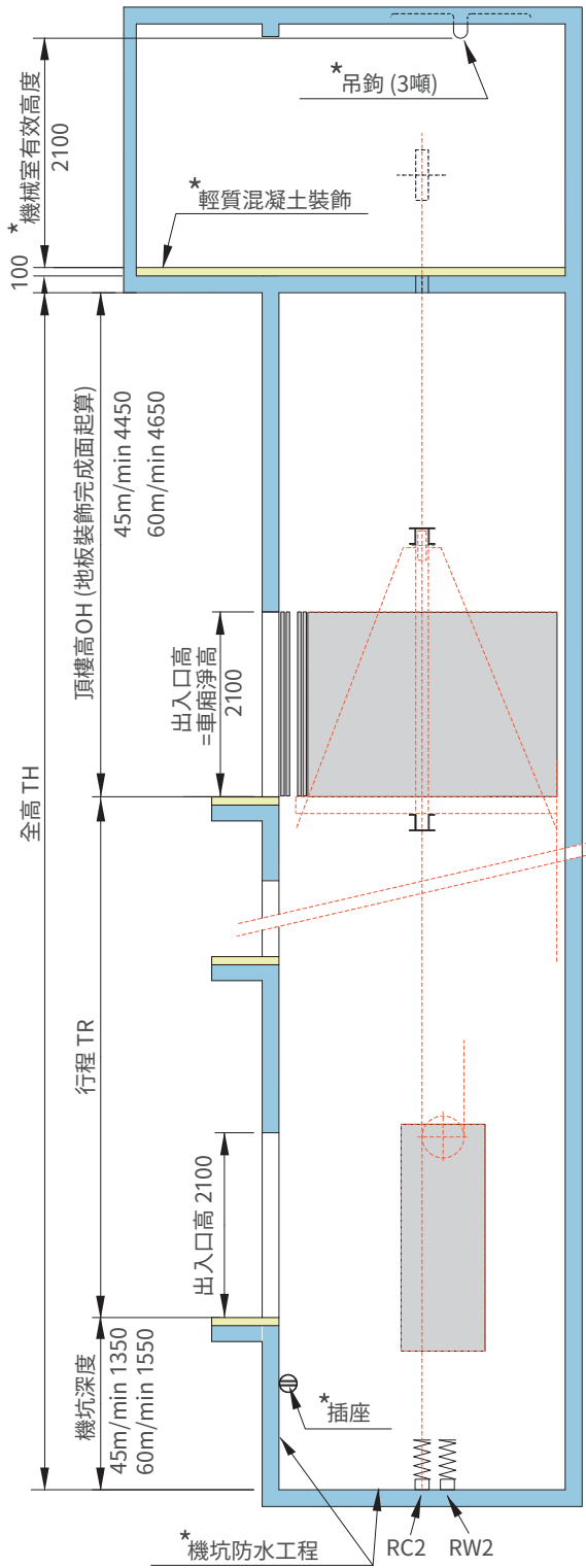
升降路立面圖
