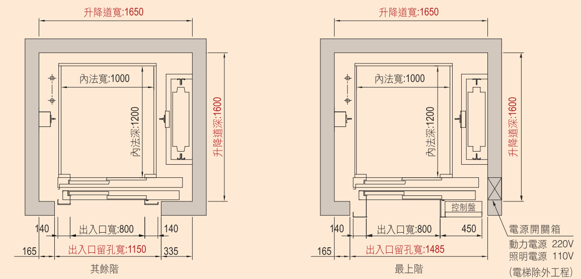
升降道平面圖
