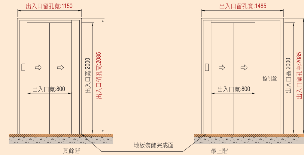
出入口示意及留孔圖
