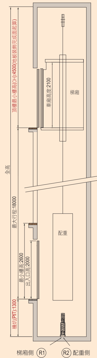
升降道斷面圖
